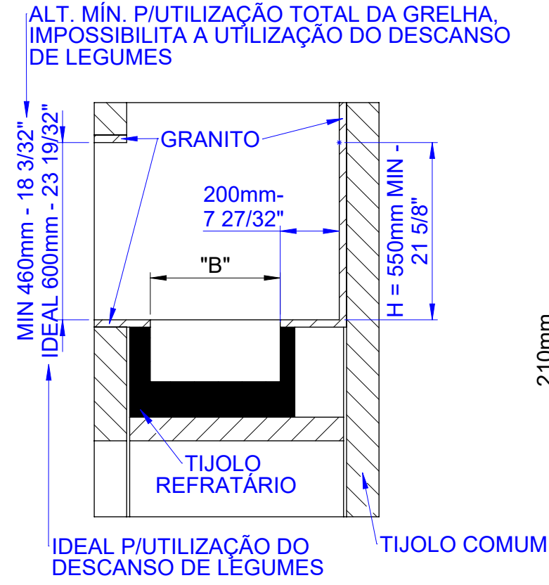
SEÇÃO A-A
