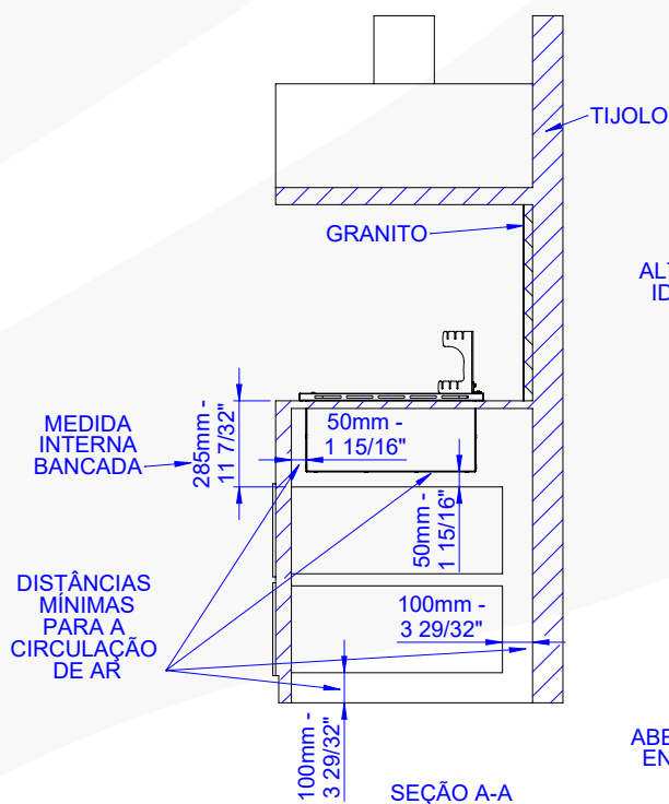
VISTA LATERAL EM CORTE
