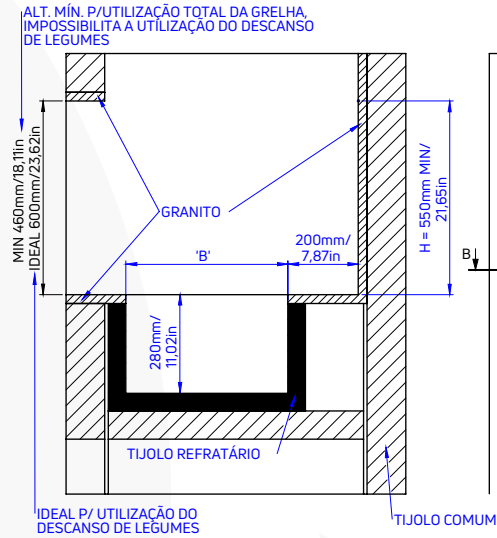
Seção A
