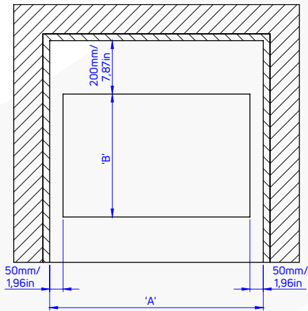
Seção B
