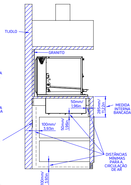
Seção A
