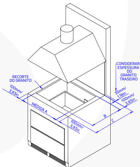
VISTA PROJETADA
