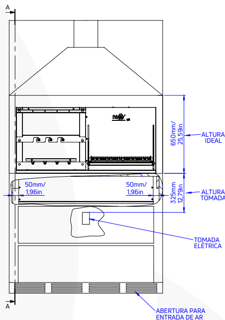
VISTA LATERAL EM CORTE
