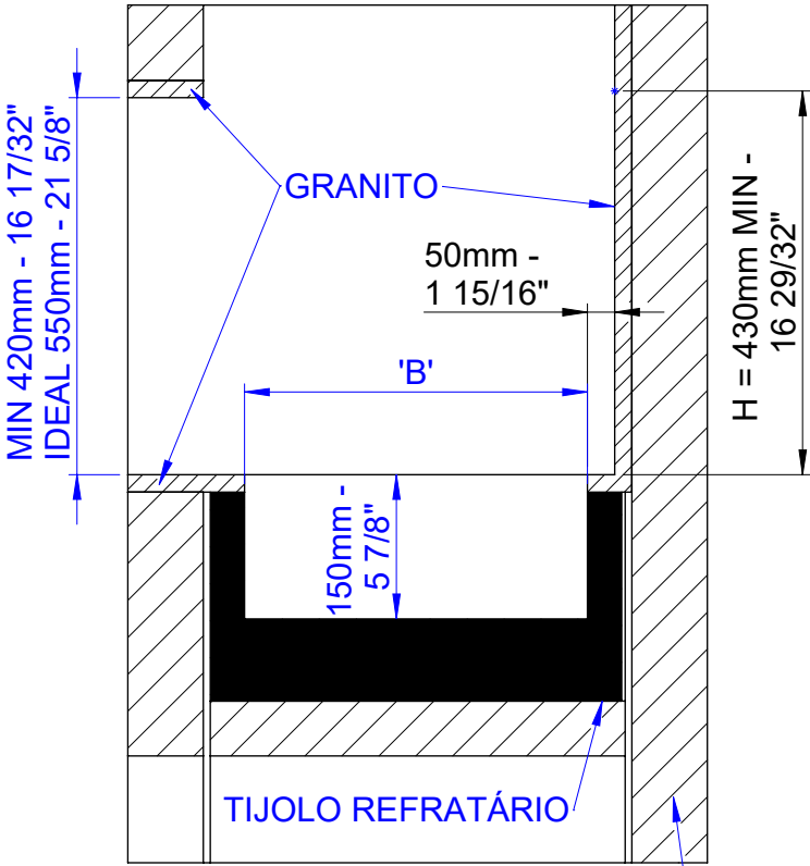
SEÇÃO A-A
