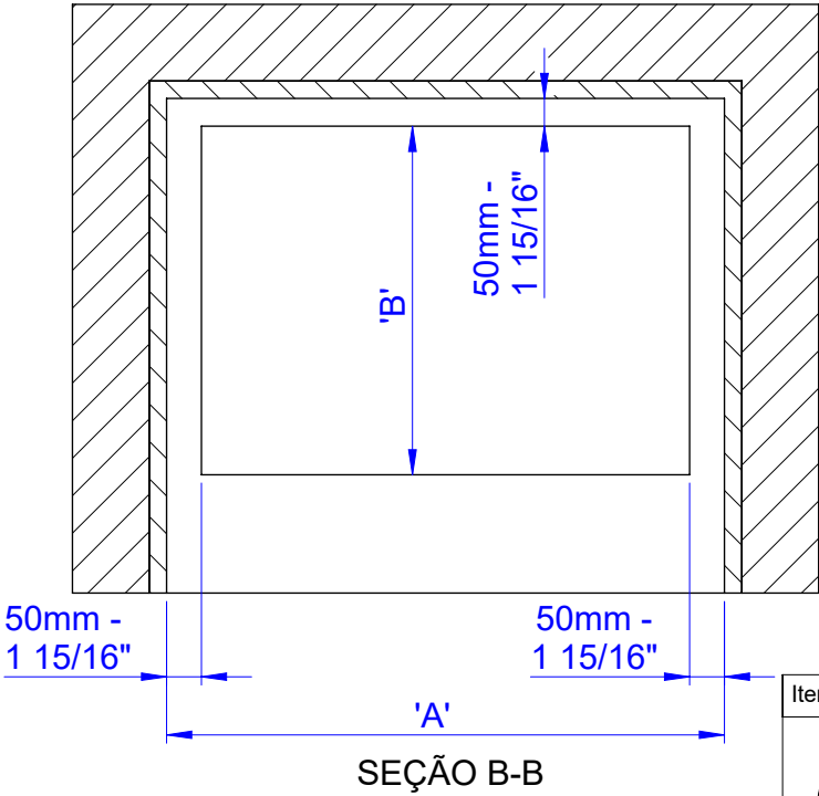
VISTA SUPERIOR EM CORTE
