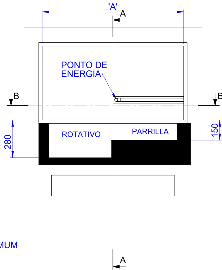
VISTA SUPERIOR EM CORTE
