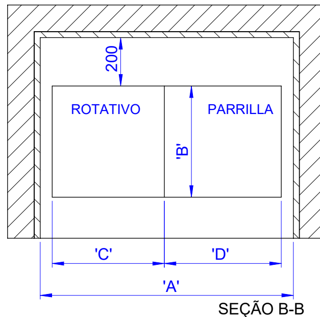
VISTA SUPERIOR EM CORTE
